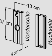
„Kabelkanal II“ L. 370 mm Art. Nr. 18955
