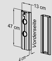
„Kabelkanal I“ L. 470 mm Art. Nr. 18950
