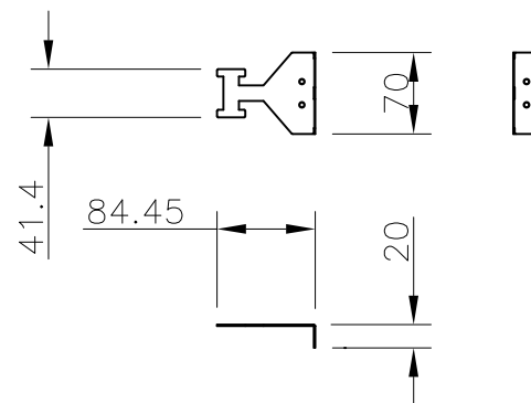
②-3 Muiti Brkt Corner & Screw set < Multi Display> (Brkt-2Ea / M4 Screw(L=8- 28Ea)
